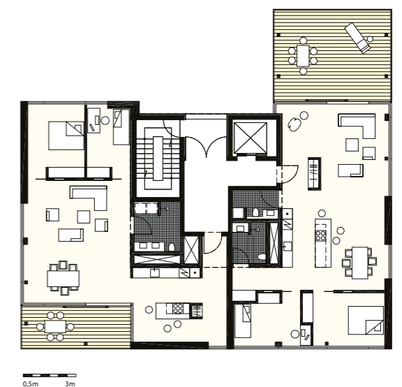
Figur 14: Konceptmodel der viser, hvordan Siloetten består af stablede elementer, der er sat uden på silokernen (øverst). Med denne opbygning er der sørget for, at alle beboere får udsigt til flere verdenshjørner. Udvikler og arkitekt kalder konceptet 'stablede parcelhuse'. Eksempel på lejlighedsplan med to altaner, 9. etage (nederst). Ideen med de store altaner er at tilbyde indflytterne et attraktivt alternativ til parcelhushaven. I Siloetten får beboerne et stort privat udeareal med en bedre udsigt end den, der er fra en parcelhushave omkranset af en hæk. De indeliggende altaner sørger samtidig for læ, god plads til ophold og til f.eks. at grille. © C.F. Møller Architects.
