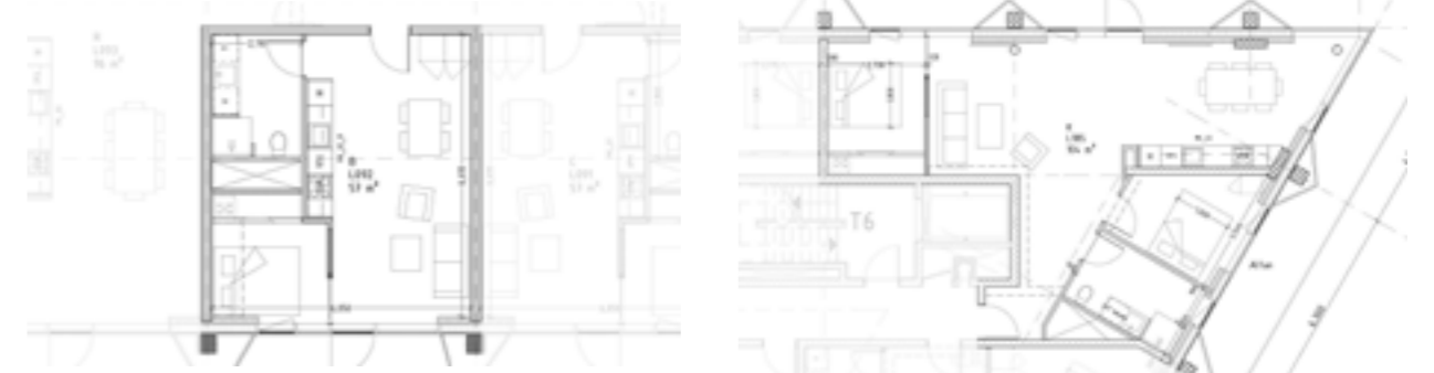
Figur 72: Lejlighedsplan for henholdsvis lille 2-rumsbolig på 58 m 2 (venstre) og en hjørnelejlighed på 3 rum på 103 m 2 (højre). © Nybolig.
